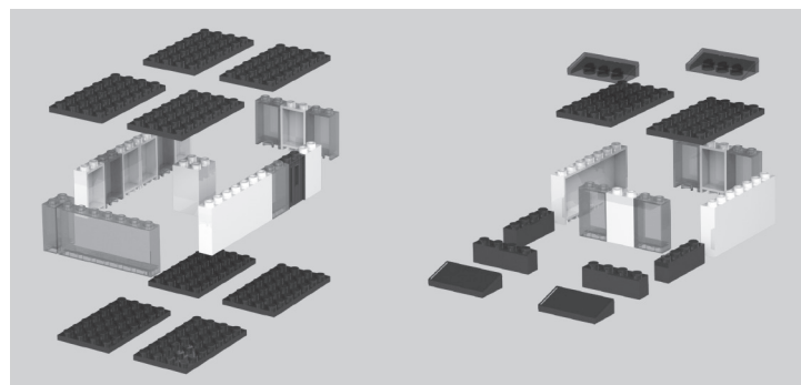
Untergeschoss
